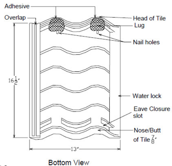
Figura 17. Reparación de Teja Rota
