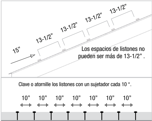
Figura 8. Instalación de Listones
