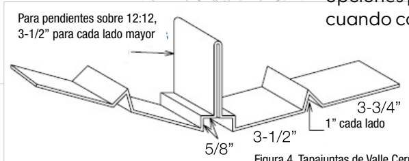
Figura 4. Tapajuntas de Valle Cerrado
