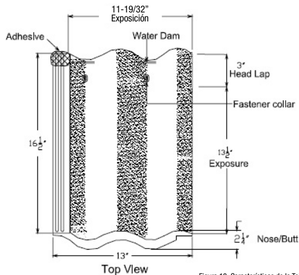
Figura 18. Características de la Teja Doble Romana
